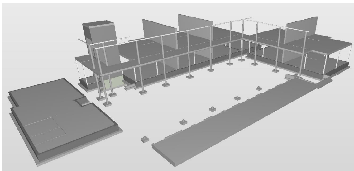
Figur 1: Betong- og stålkonstruksjon
